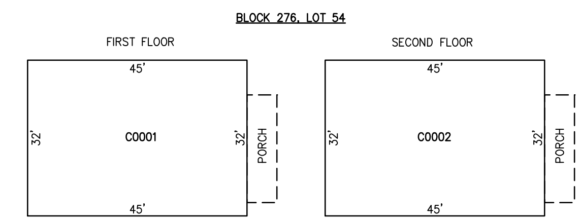
DETAILS SCALE: 1"=20'
