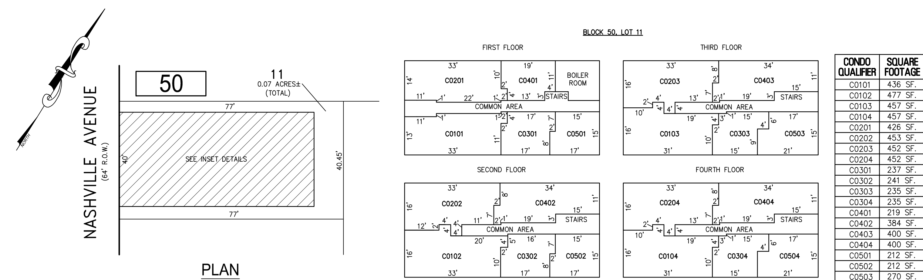
DETAILS SCALE: 1"=20'
