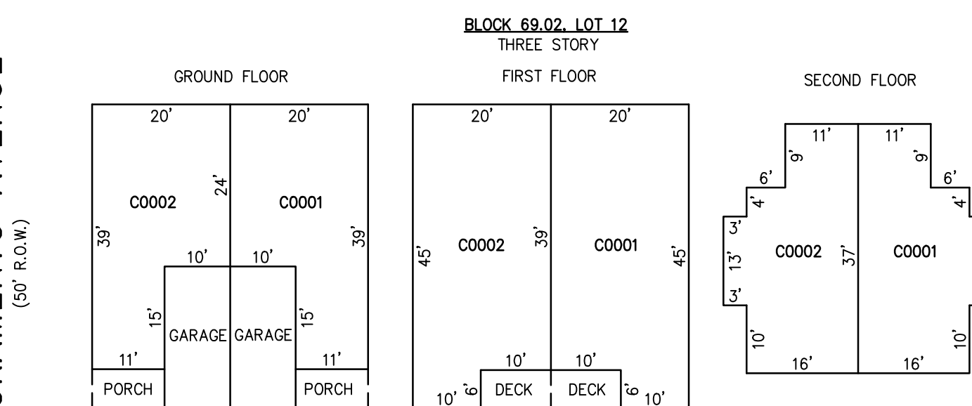
DETAILS SCALE: 1"=20'
