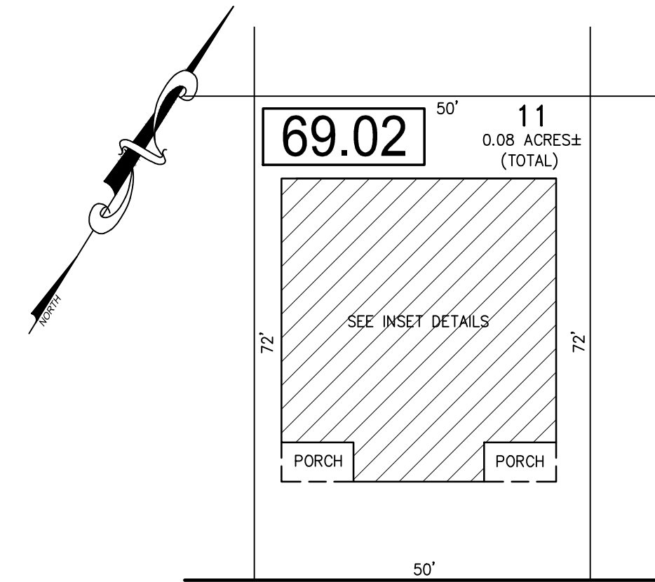
PLAN SCALE: 1"=20'
