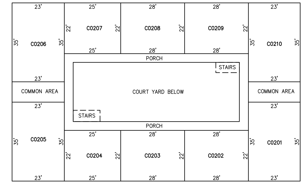
DETAILS SCALE: 1"=20'
