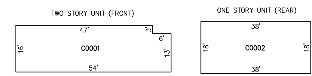
DETAILS SCALE: 1"=20'
